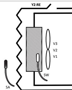
2 TUBI + RESISTENZA ELETTRICA PER IL CALDO IN SOSTITUZIONE/INTEGRAZIONE + VALVOLA 3 VIE
