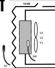
2 TUBI SOLO FREDDO + RESISTENZA ELETTRICA PER IL CALDO
