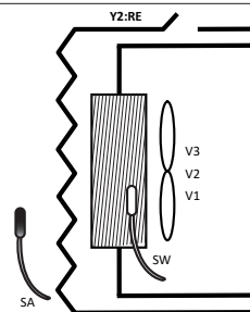
2 TUBES + RÉSISTANCE ÉLECTRIQUE POUR LE CHAUD EN REMPLACEMENT/INTÉGRATION + VANNE 3 VOIES
