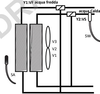
4 TUBI CON VALVOLE A 3 VIE
