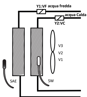
4 TUBI CON VALVOLE A 2 VIE
