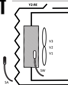
2 TUBES FROID SEUL + RÉSISTANCE ÉLECTRIQUE POUR LE CHAUD
