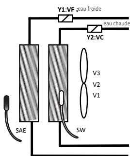
4 TUBES AVEC VANNES 2 VOIES
