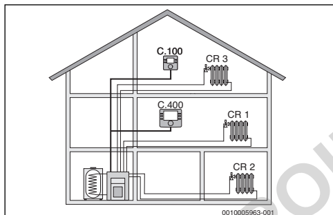
Fig. 2 Esempio per impianto di riscaldamento con tre circuiti di riscaldamento e CR 100 come termoregolatore di zona (abitazione unifamiliare con appartamento con entrata separata o officina)
