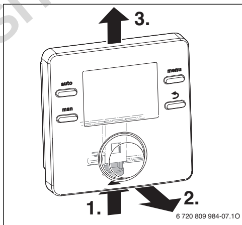
Fig. 10 Rimozione del termoregolatore
