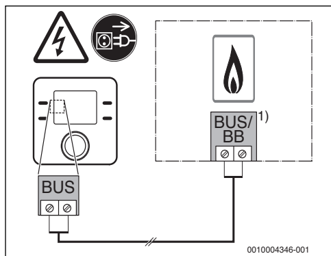
Fig. 8 Collegamento di un termoregolatore al generatore di calore
