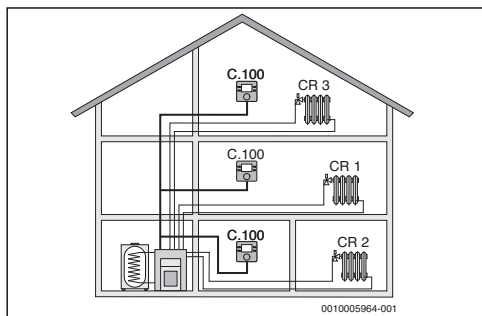
Fig. 3 Esempio per impianto di riscaldamento con tre circuiti di riscaldamento, ciascuno di essi dotato di un C 100 come termoregolatore (casa plurifamiliare)
