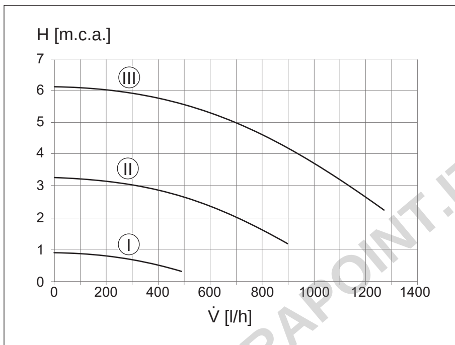
Curve caratteristiche del circolatore di serie in GC2300W 24 C e GC2300W 24/30 C
