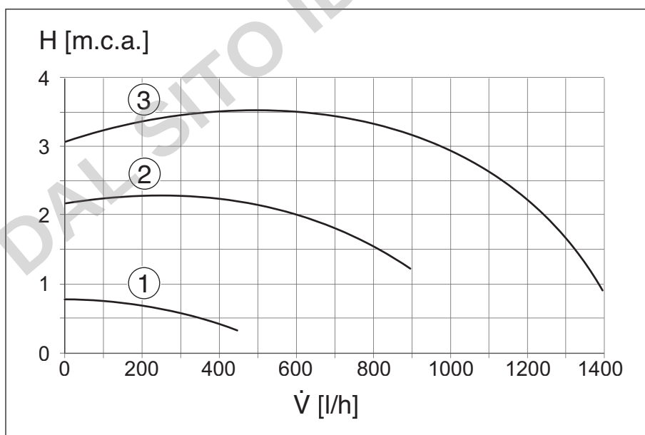
Curve caratteristiche del circolatore di serie in GC2300W 24 C e GC2300W 24/30 C
