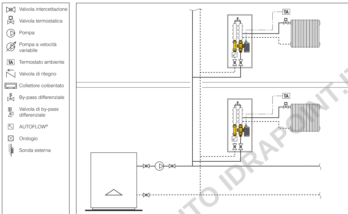
Impianto con valvole di zona a due vie e valvola di sfioro.
