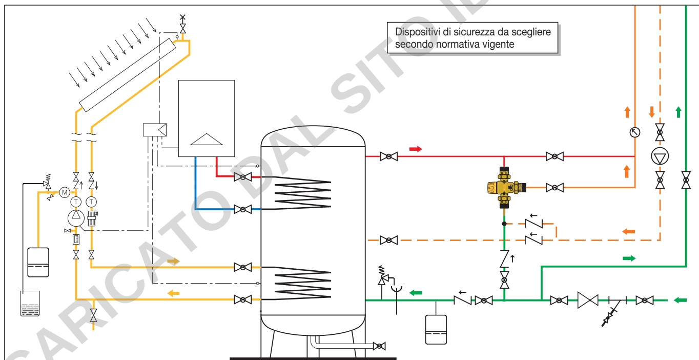
Impianto con integrazione termica a circolazione forzata
