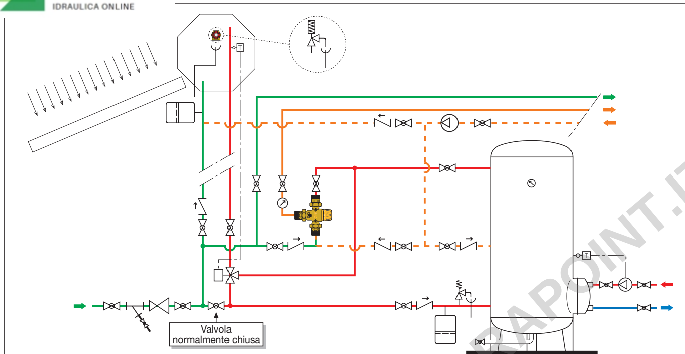
Impianto con integrazione termica a circolazione forzata
