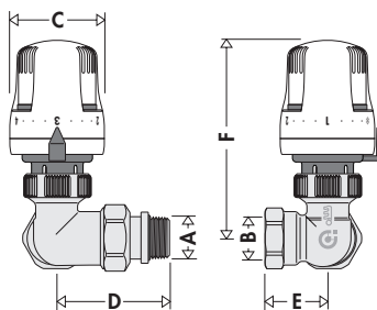
Versione Destra
