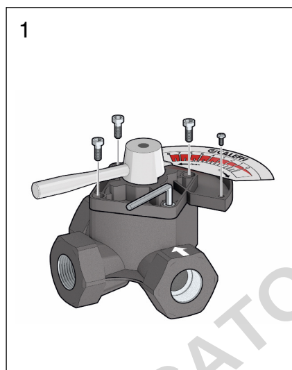
Esempio di installazione valvola a 3 vie a settore serie 612 con funzione miscelatrice
