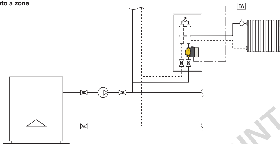
Impianto a zone
