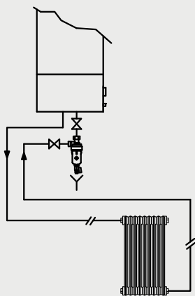
Schema di installazione
