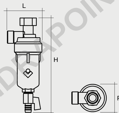
Misure di ingombro
