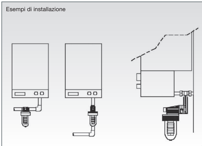
Disegni di ingombro
