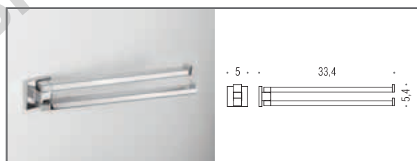
B3712 ○ Porta salvietta doppio a snodo Double bar towel holder
