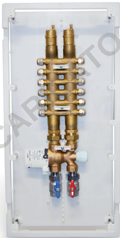
Fig.6 - Esempio installazione valvola di zona (Serie 561T + attuatore Serie 580T) in cassetta di ispezione Serie 824M.
