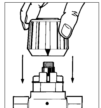
Fig.3 Reinserire il volantino in modo che il riferimento a V corrisponda al rilievo sul corpo. In questa posizione il volantino è bloccato.
