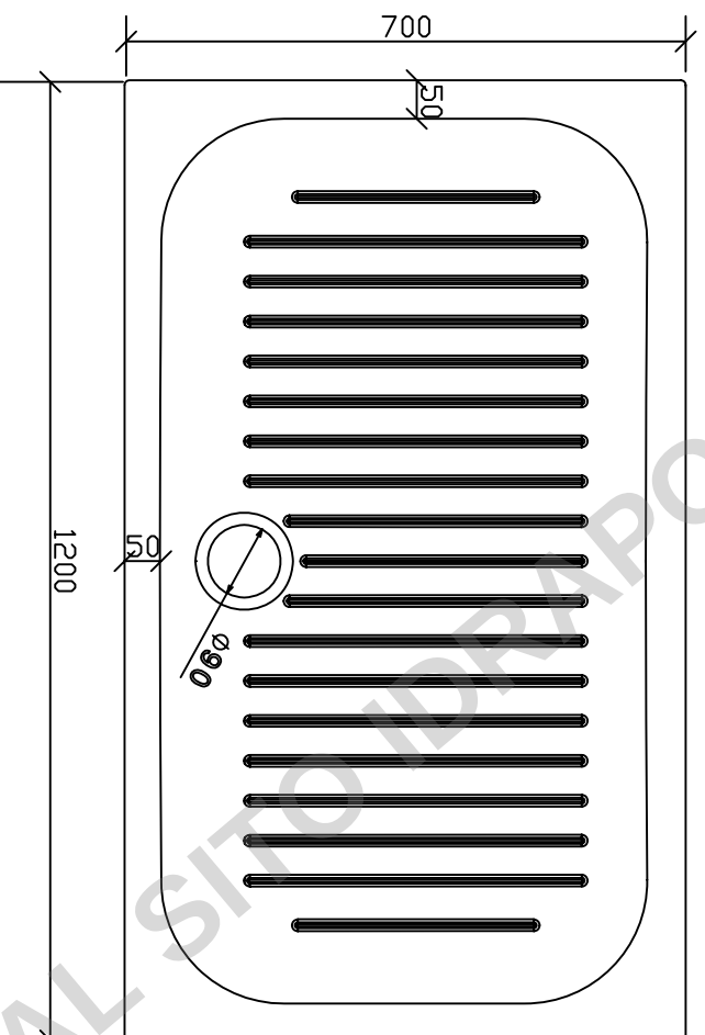
Vista dall'alto
