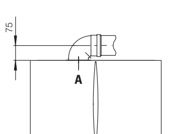
Quota kit concentrico Ø 60/100
