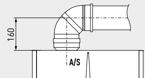
Quota kit concentrico Ø 80/125
