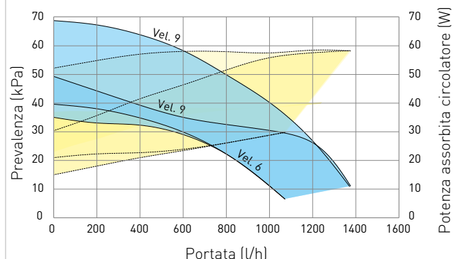
Grafico portata e prevalenza VICTRIX ZEUS SUPERIOR 30/35
