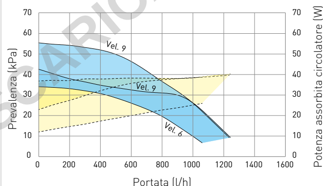
Grafico portata e prevalenza VICTRIX ZEUS SUPERIOR 25
