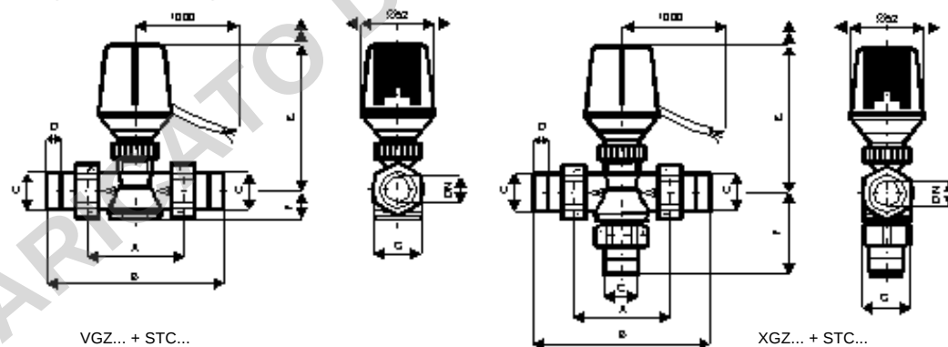
VGZ... + STC...
